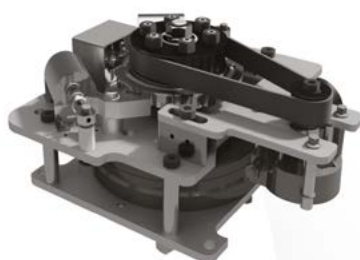
Drehkreuzmechanismus – hochwertige Bremse mit kurzer Ansprechzeit.
